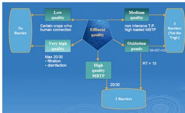
圖 3. 再生水水質與所需屏障數的關係。
