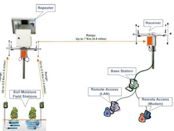
◆圖 1. 以色列管路灌溉控制系統。 右上圖為模式圖，左下圖 為實際應用裝置。
