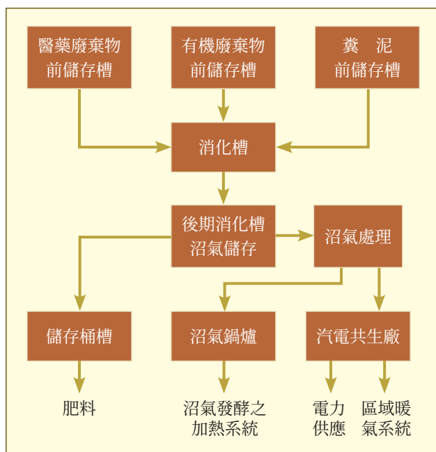
圖 2. Lintrup 鎮的集中式沼氣工廠之操作流程
