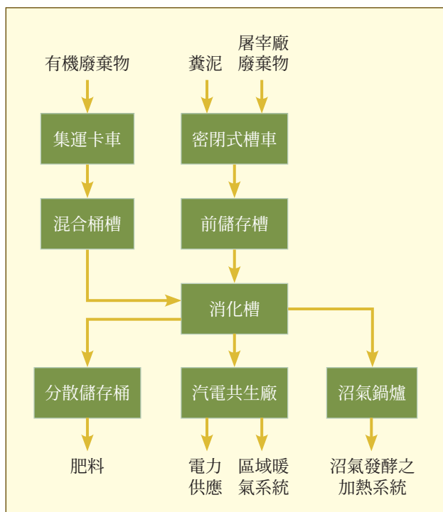
圖 1. Ribe 鎮的集中式沼氣工廠之操作流程
